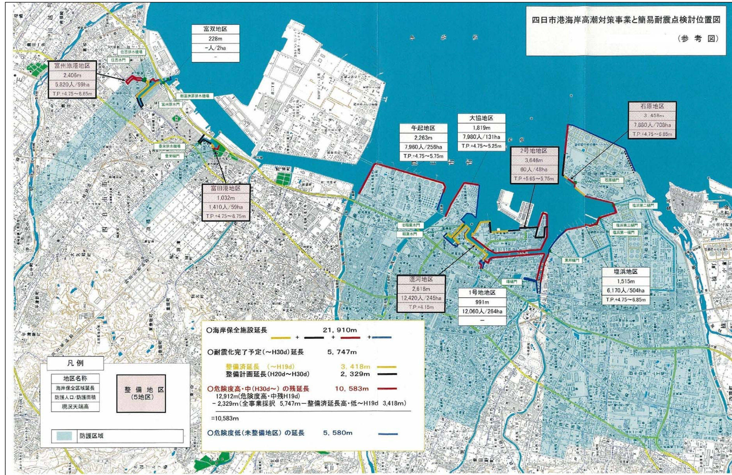
図 6.2.7 四日市港の海岸保全施設と耐震点検結果
