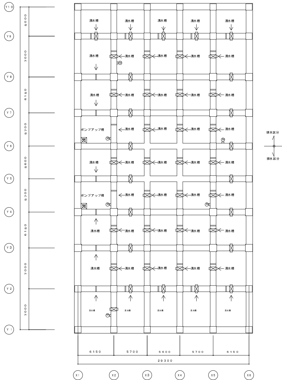
基礎建レベル平面図
